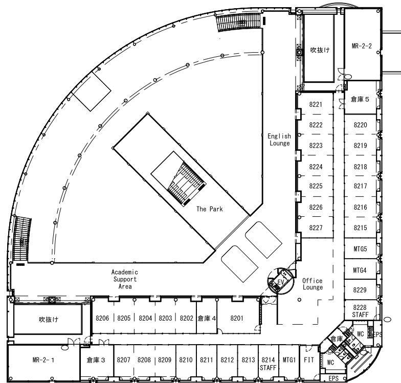
2階平面図
