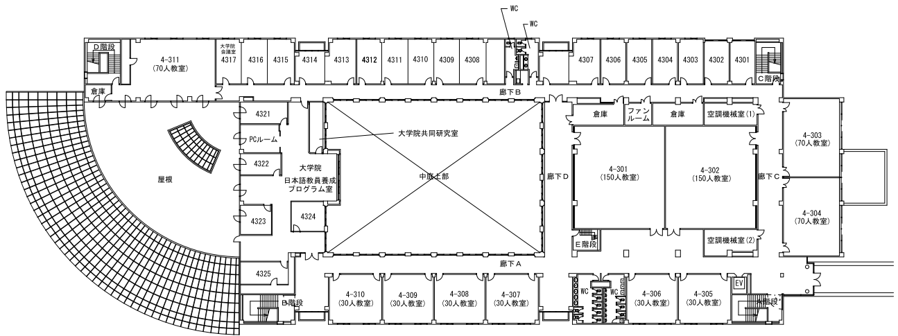
3階平面図
