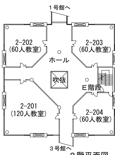
2階平面図
