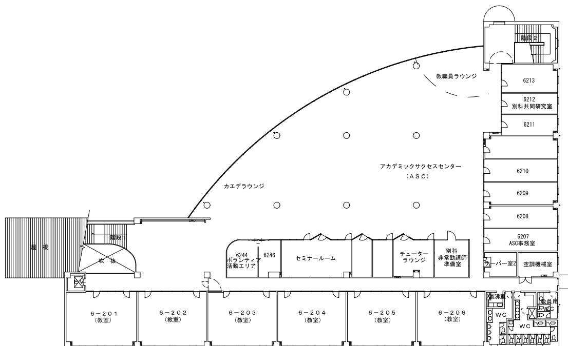
2階平面図
