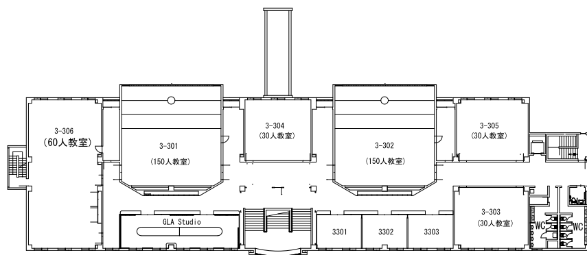
3階平面図
