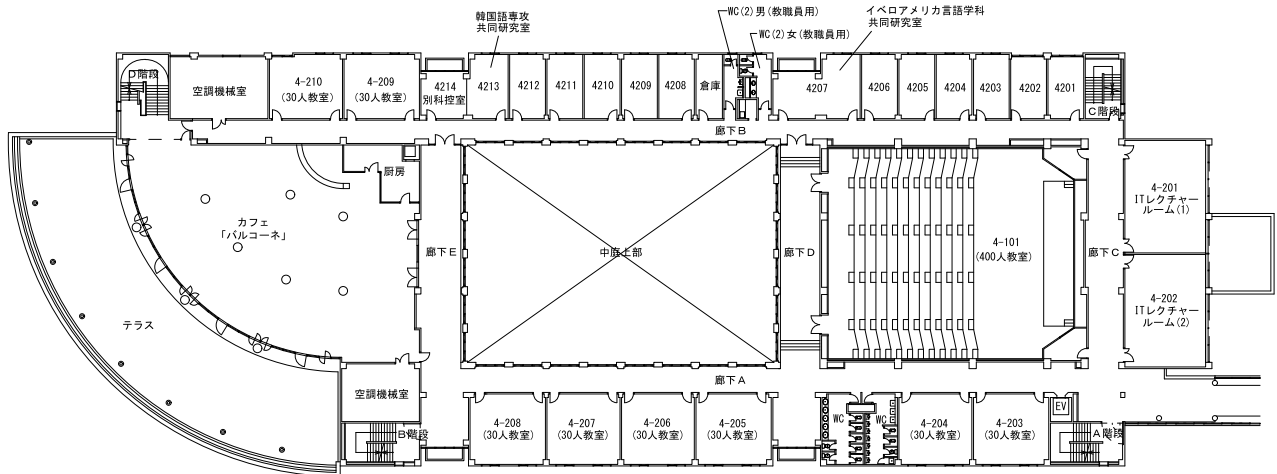
2階平面図
