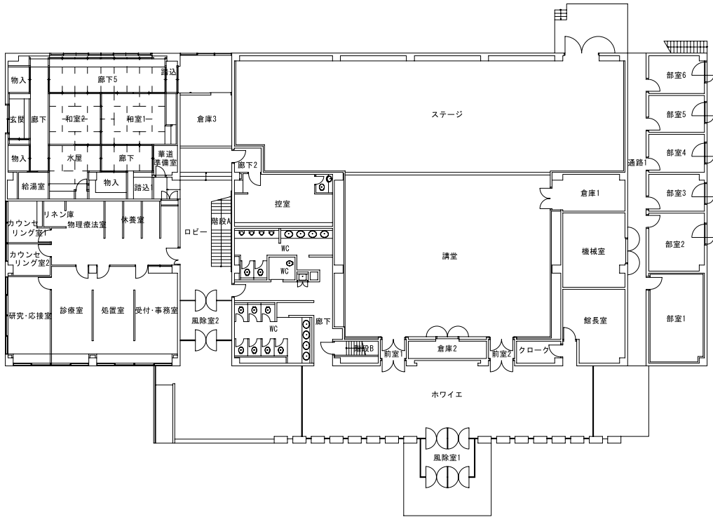
1階平面図
