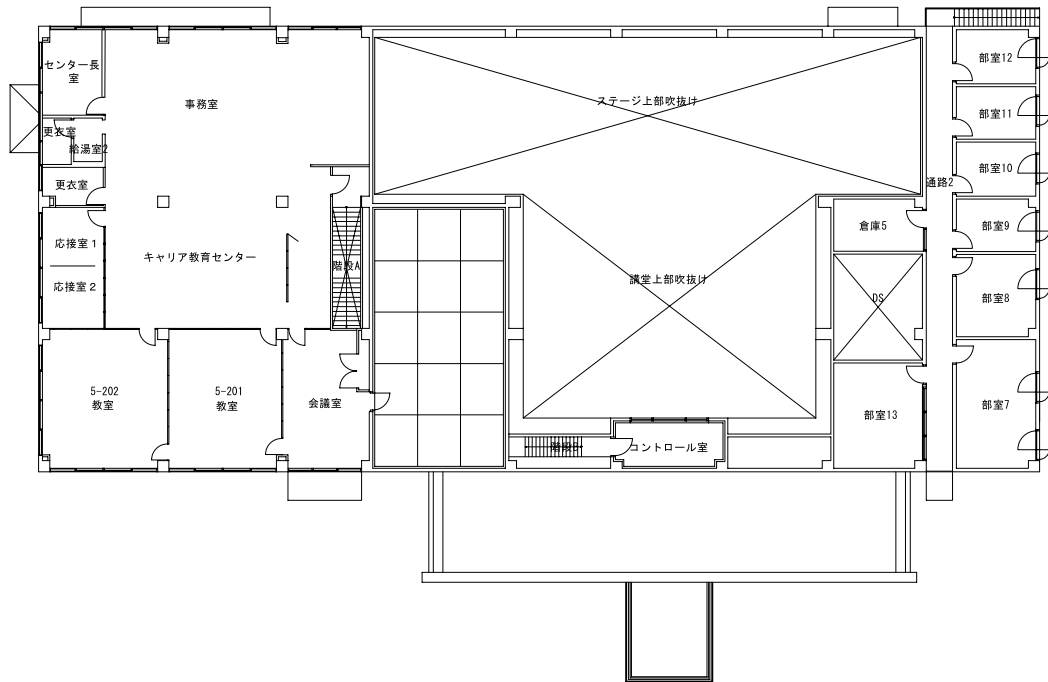
2階平面図
