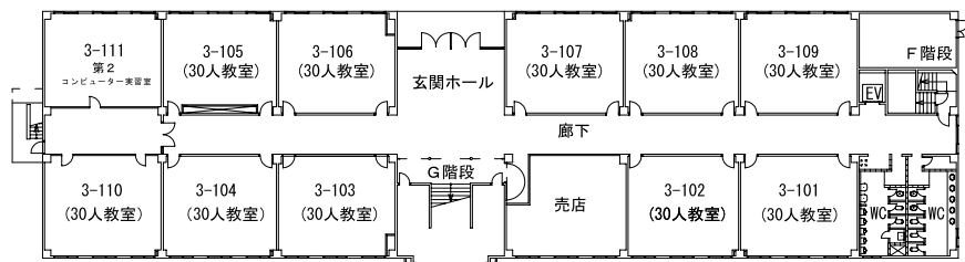
1階平面図
