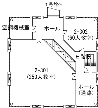
3階平面図
