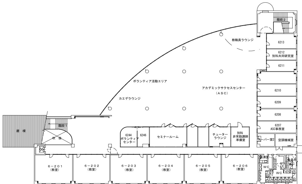
2 階平面図
