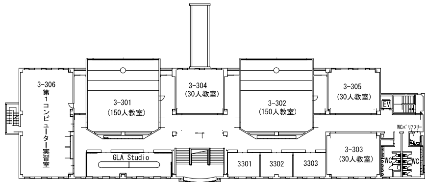
3階平面図
