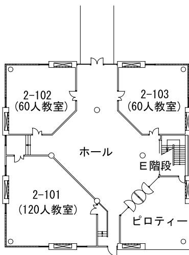
1階平面図
