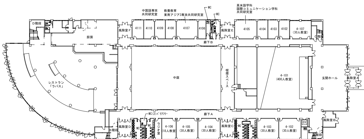
1階平面図
