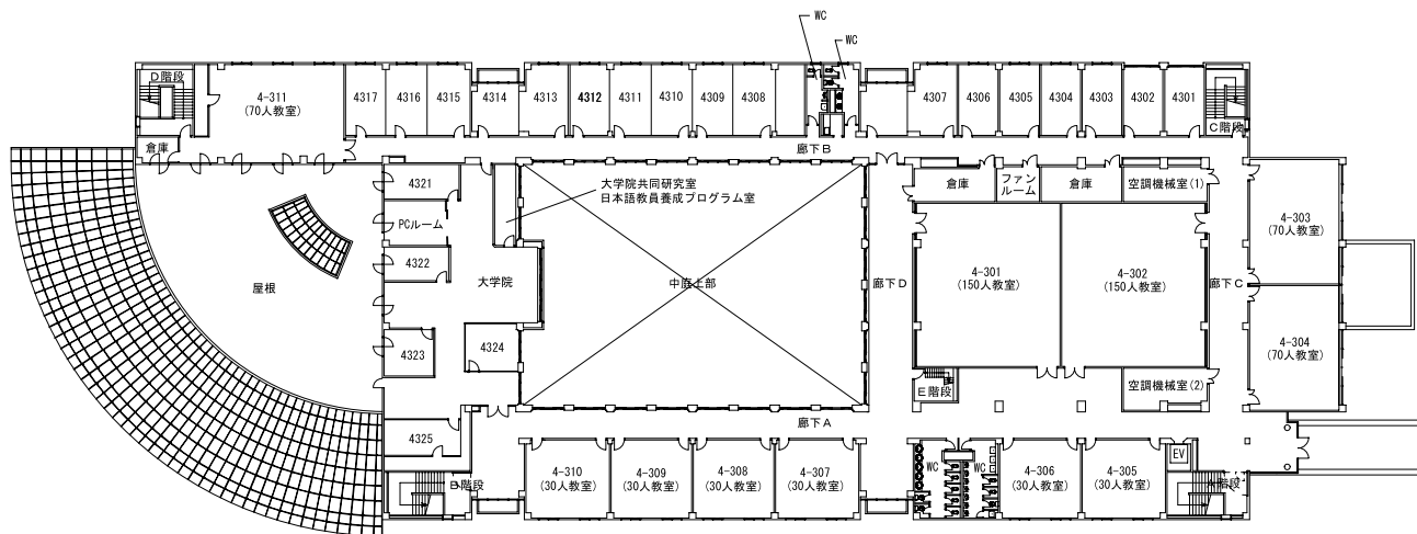
3階平面図
