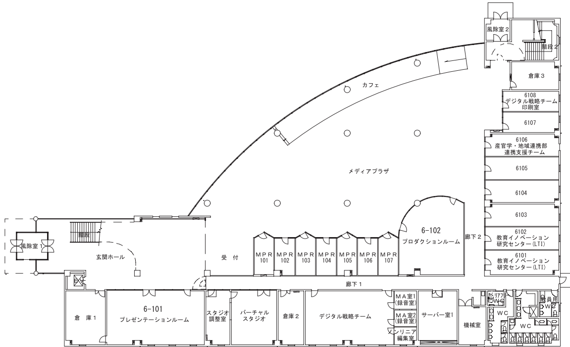
1 階平面図
