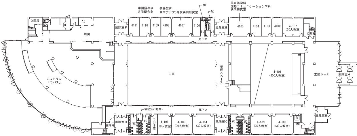
1 階平面図
