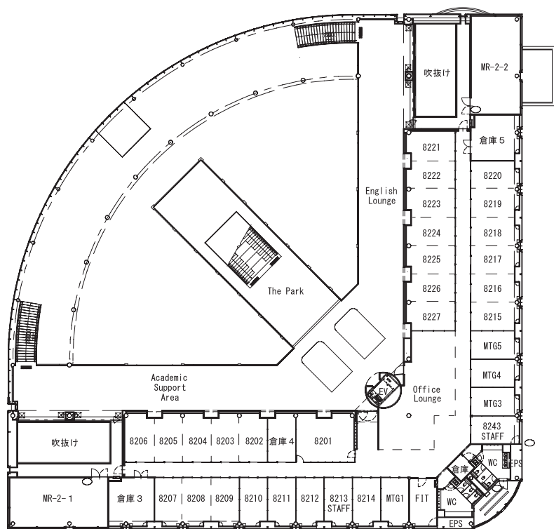
2階平面図
