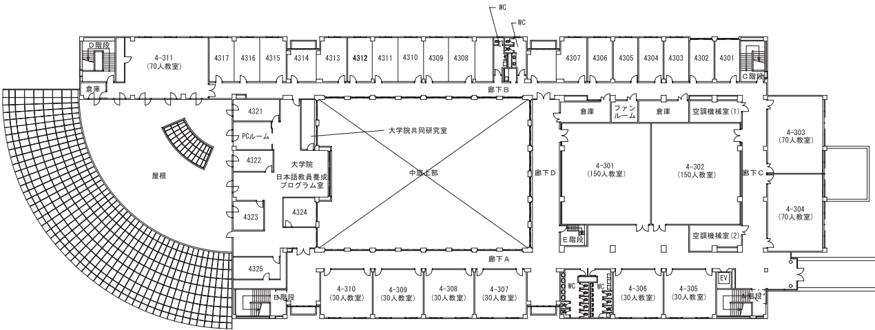
3 階平面図
