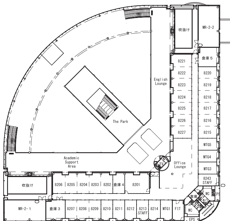
2階平面図
