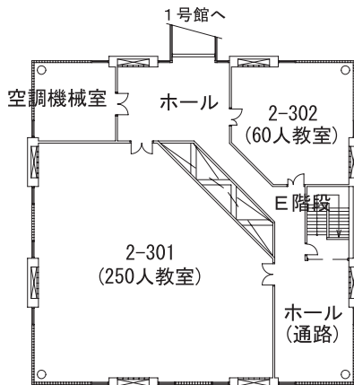
3階平面図
