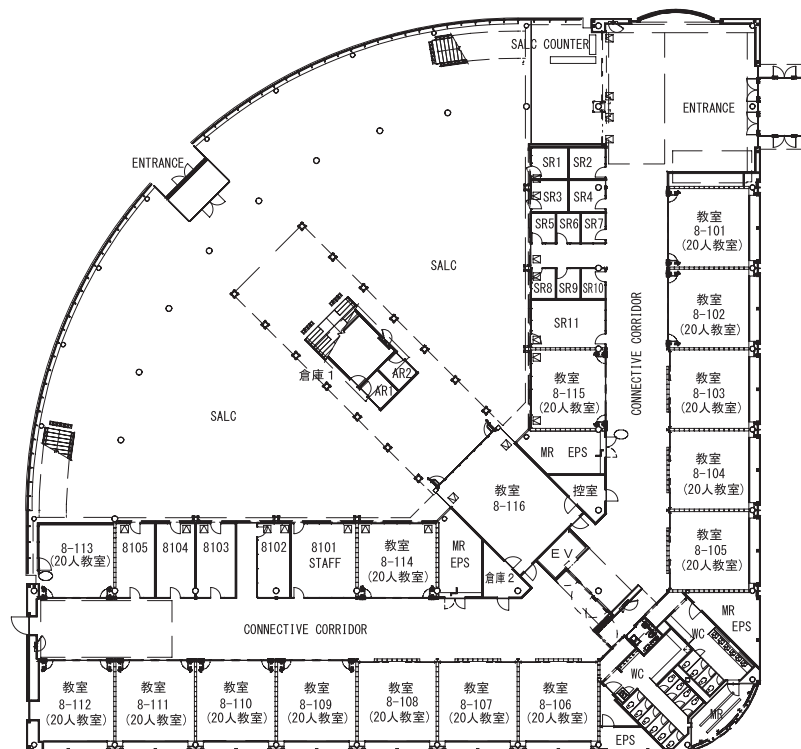
1階平面図
