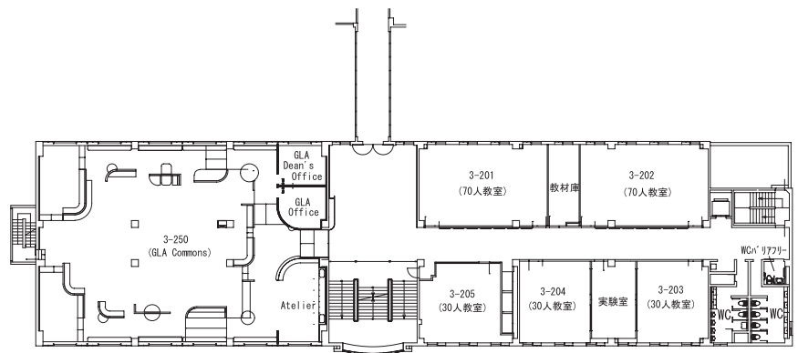
2階平面図
