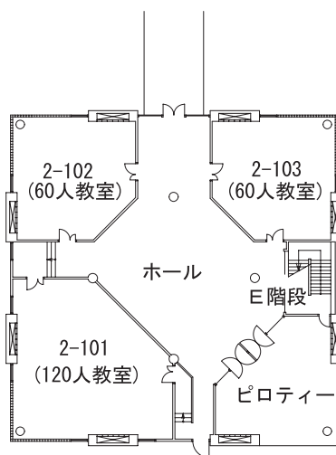
1階平面図
