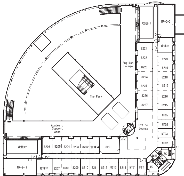
2階平面図
