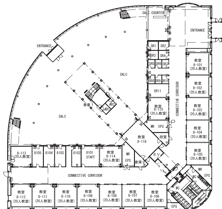
1階平面図
