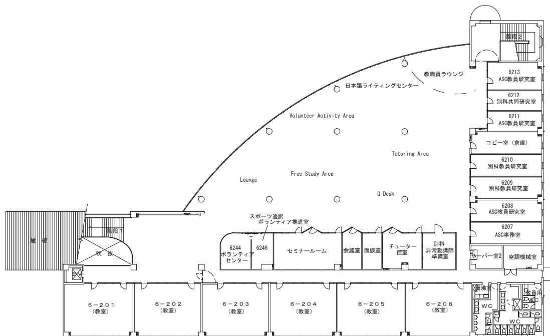
2 階平面図
