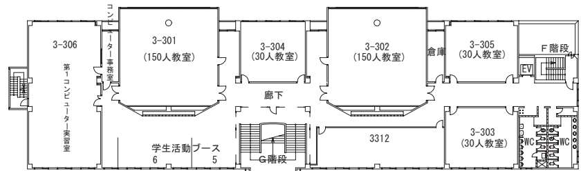
3階平面図
