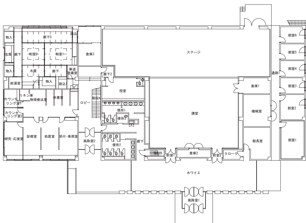
1階平面図
