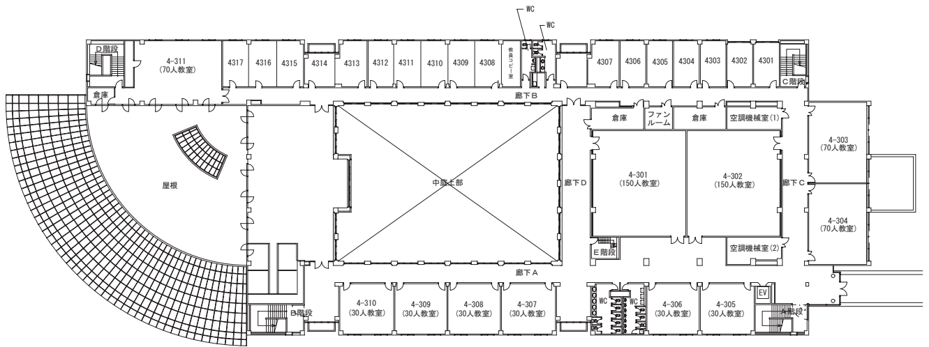
3階平面図
